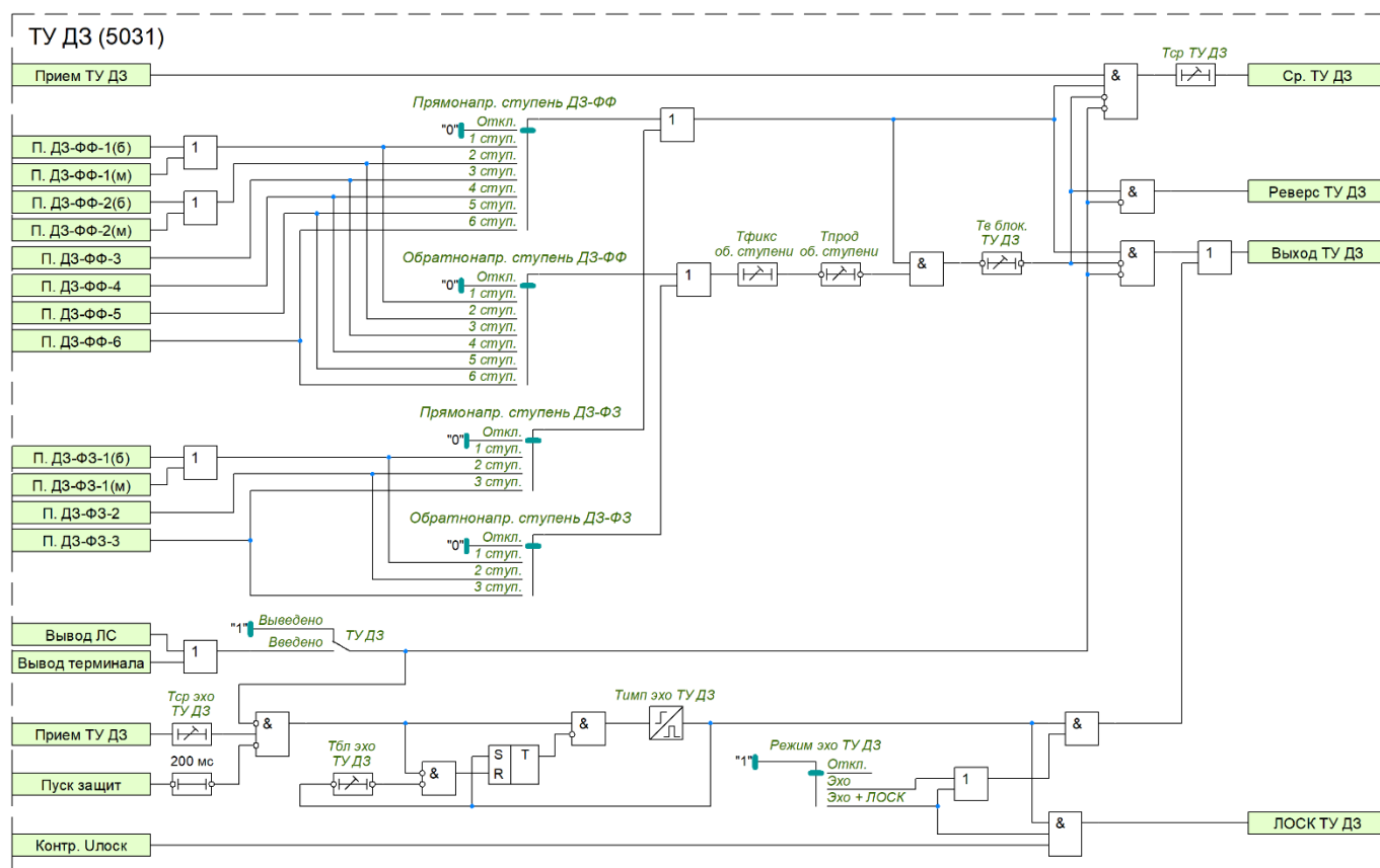
Рисунок 36 – Функциональная схема ТУ ДЗ
