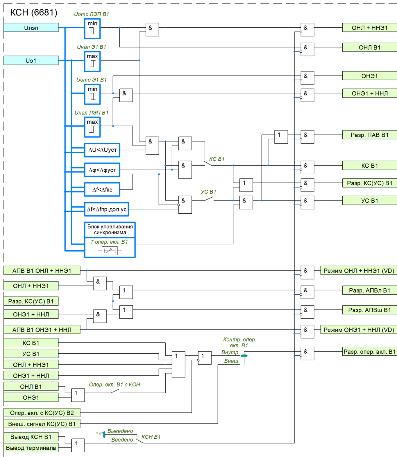
Рисунок 41 – Функциональная схема КСН В1
