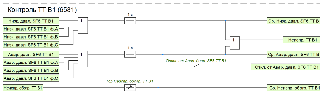
Рисунок 48 – Функциональная схема контроля ТТ В1
