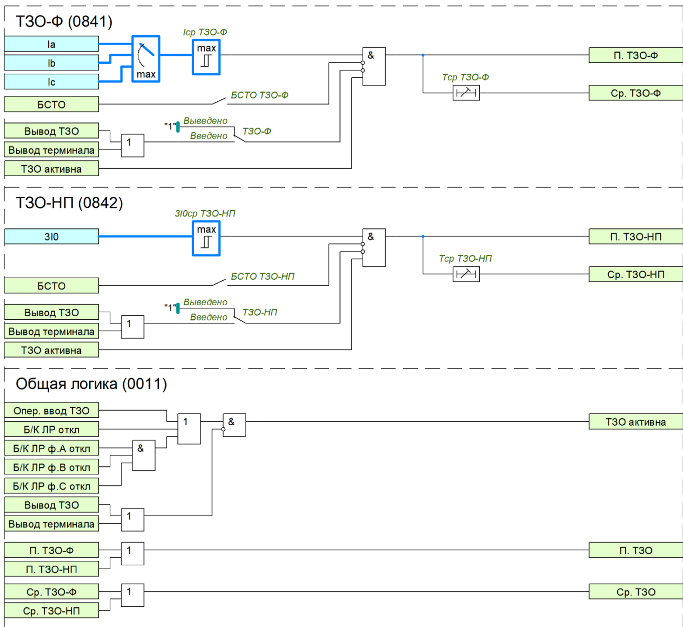
Рисунок 28 – Функциональная схема ТЗО
