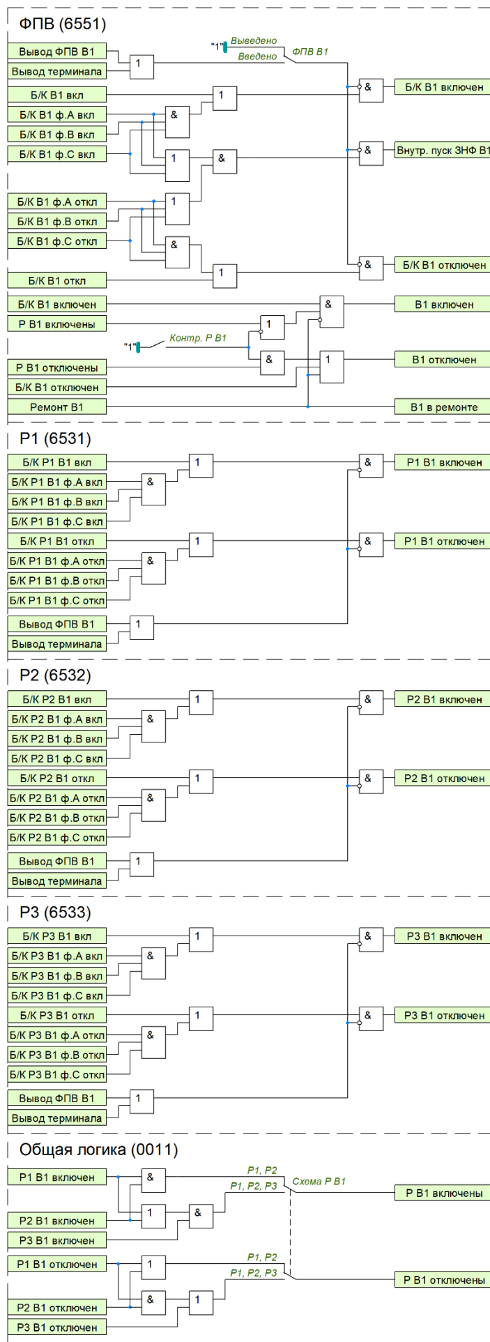
Рисунок 56 – Функциональная схема ФПВ В1
