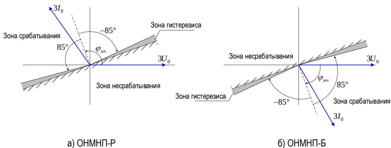
Рисунок 19 – Характеристики срабатывания ОНМНП
