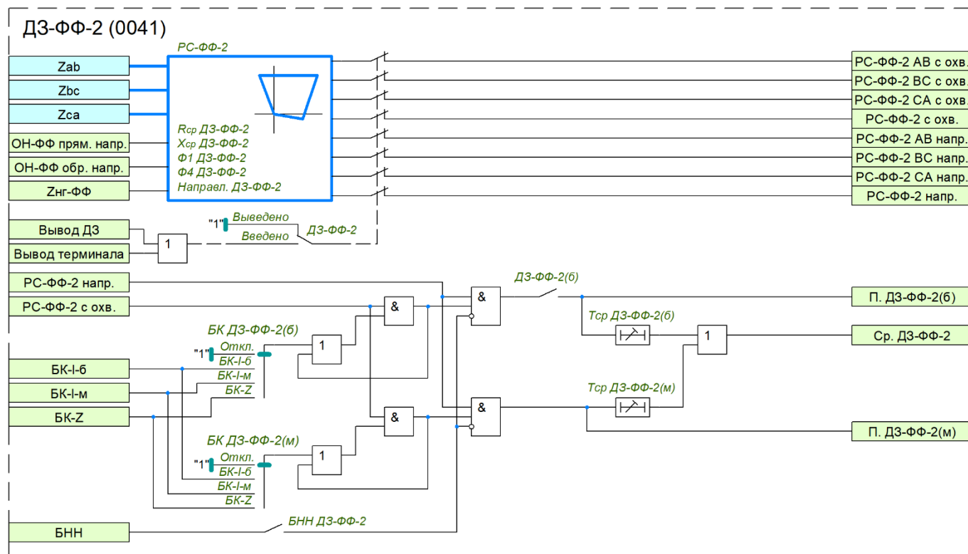
Рисунок 8 – Функциональная схема ДЗ-ФФ-2
