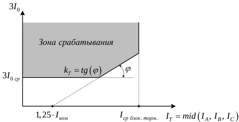
Рисунок 6 – Характеристика срабатывания ИО 3I0 ООВП
