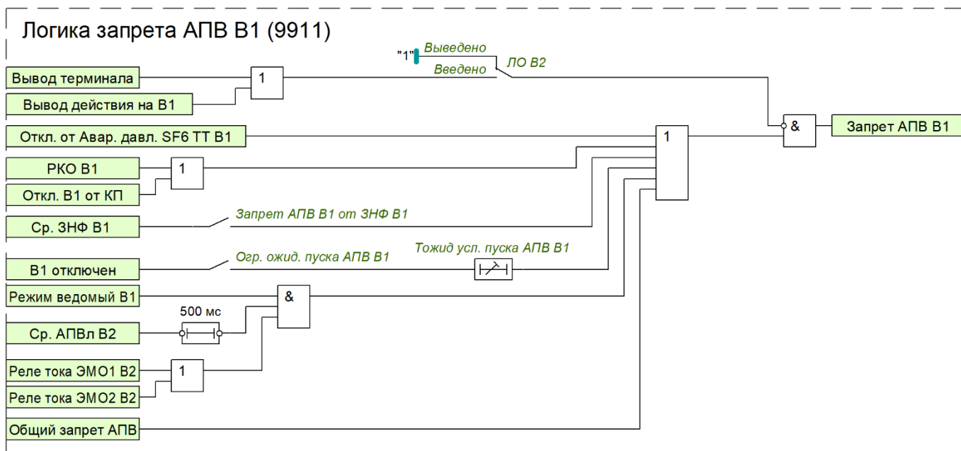
Рисунок 45 – Функциональная схема запрета АПВ В1
