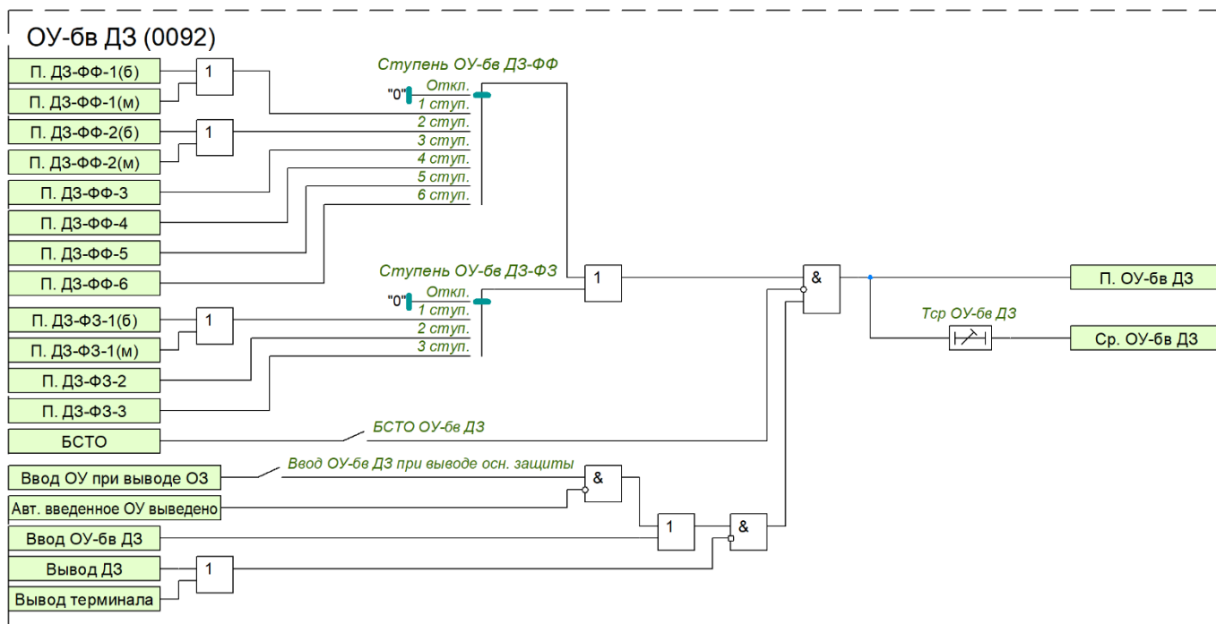
Рисунок 14 – Функциональная схема ОУ-бв ДЗ
