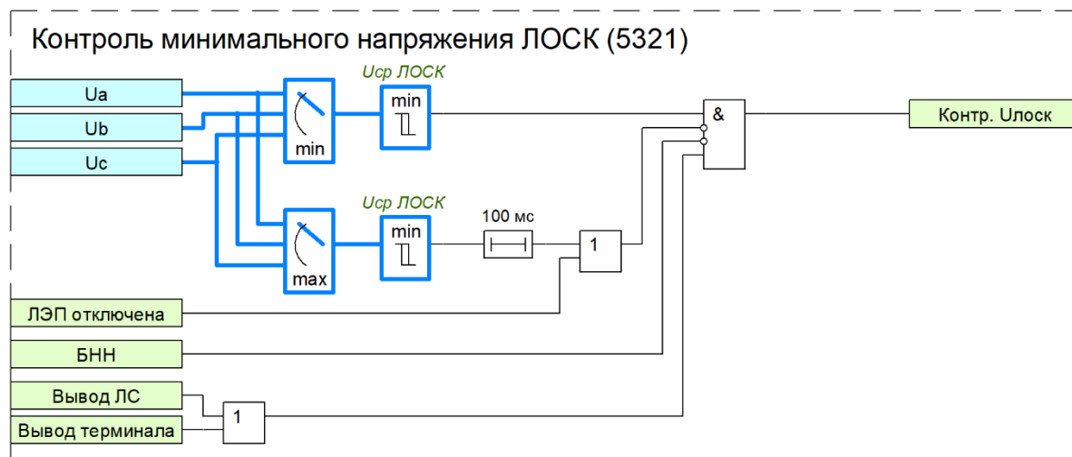
Рисунок 38 – Функциональная схема контроля минимального напряжения ЛОСК
