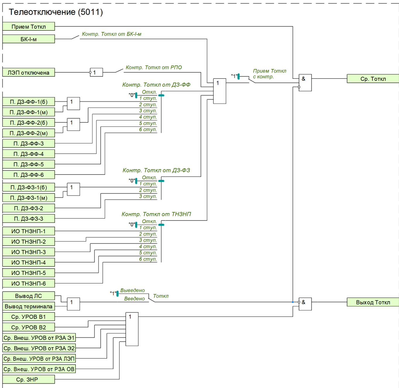
Рисунок 34 – Функциональная схема Тоткл
