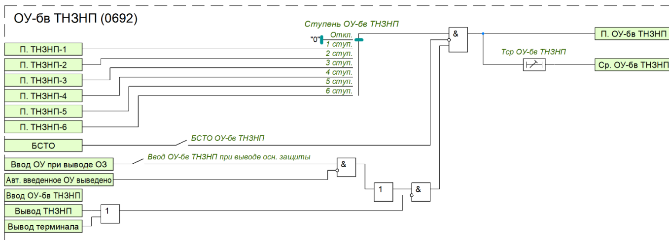
Рисунок 22 – Функциональная схема ОУ-6в ТНЗНП
