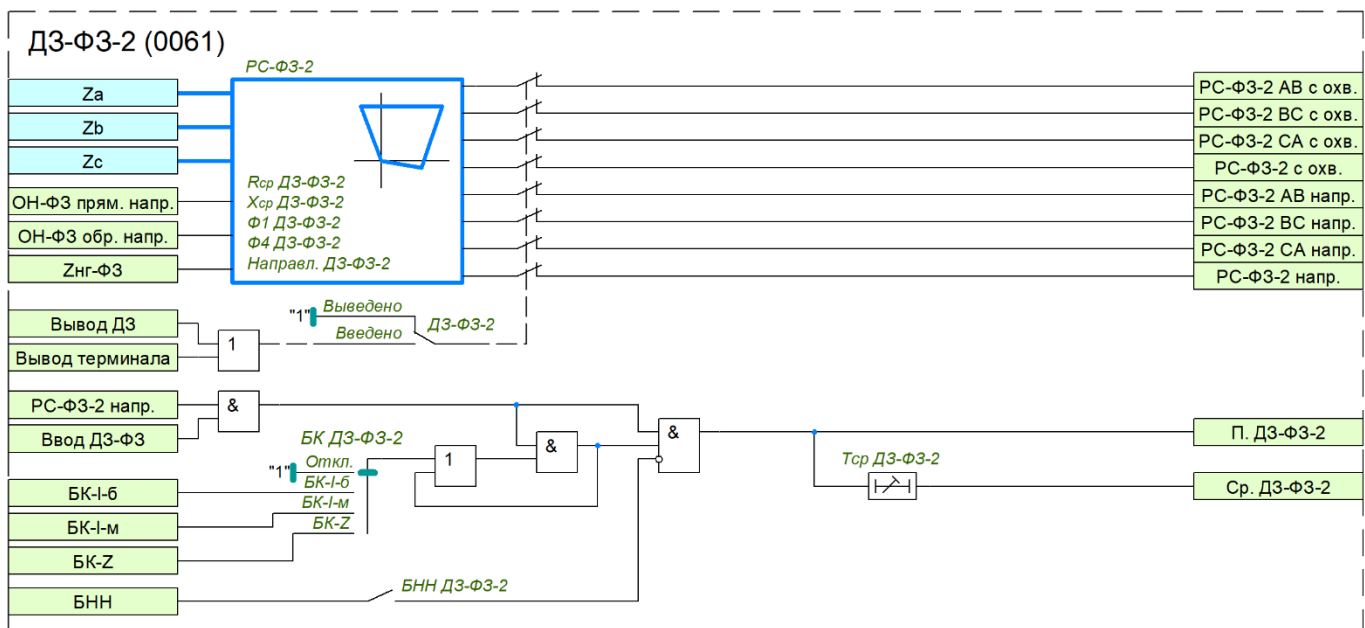
Рисунок 11 – Функциональная схема ДЗ-ФЗ-2
