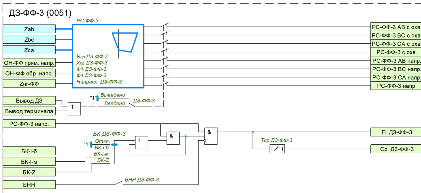
Рисунок 9 – Функциональная схема ДЗ-ФФ-3
