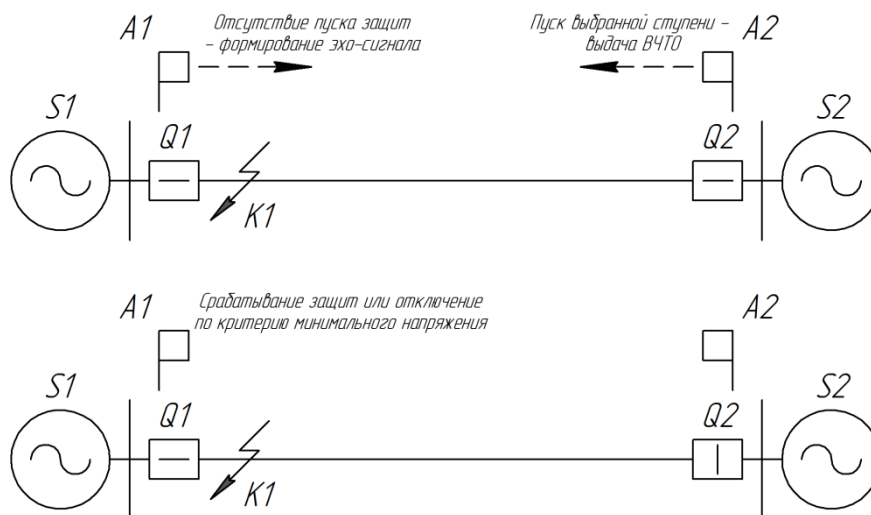
Рисунок 37 – Пояснение к принципу действия эхо-логики
