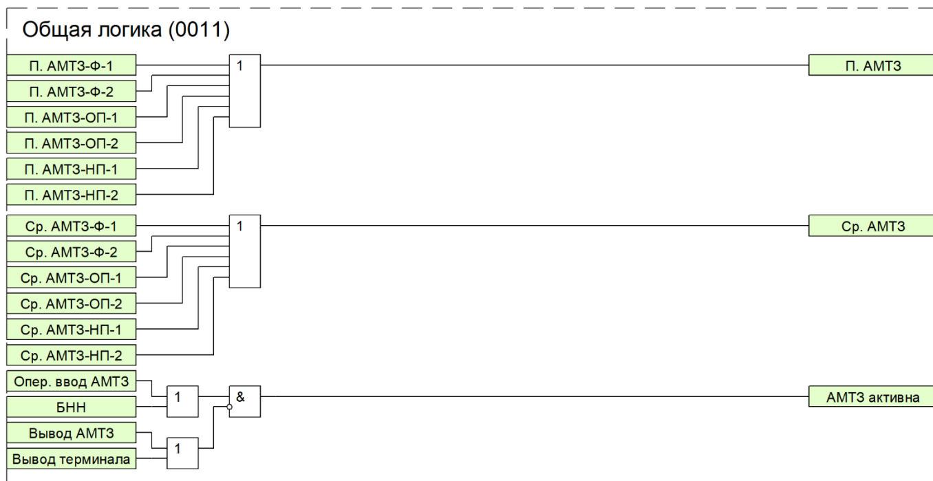
Рисунок 27 – Функциональная схема общей логики АМТЗ
