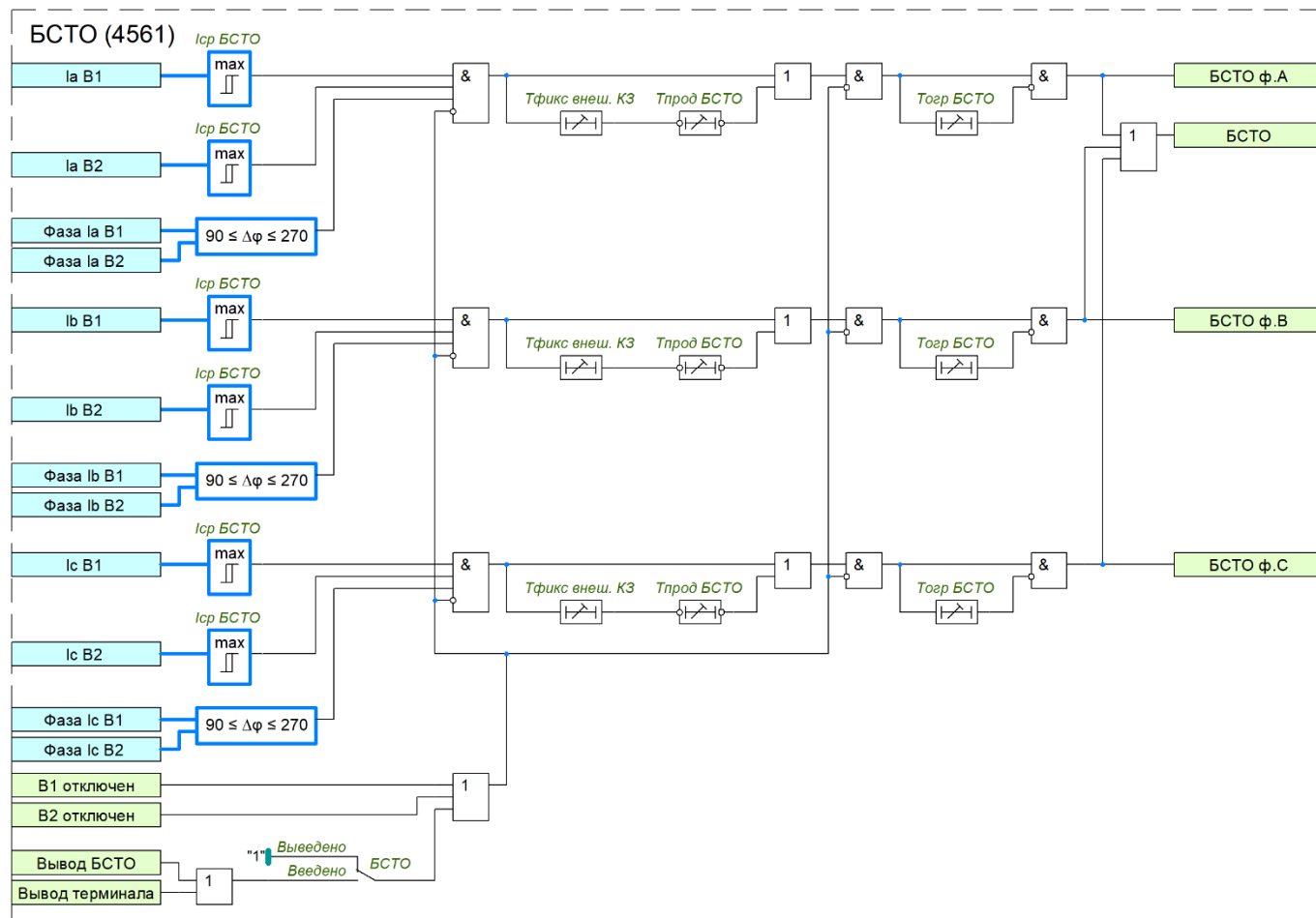
Рисунок 29 – Функциональная схема БСТО
