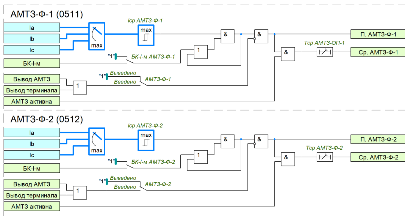
Рисунок 26 – Функциональная схема ступеней АМТЗ-Ф
