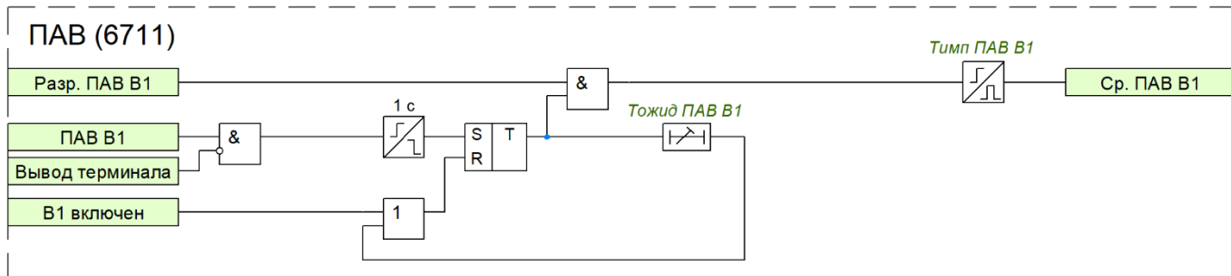
Рисунок 46 – Функциональная схема ПАВ В1
