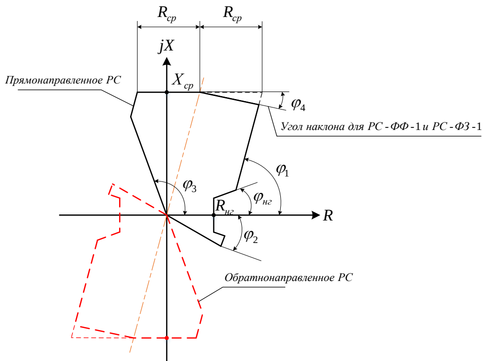
Рисунок 4 – Характеристики срабатывания направленного РС
