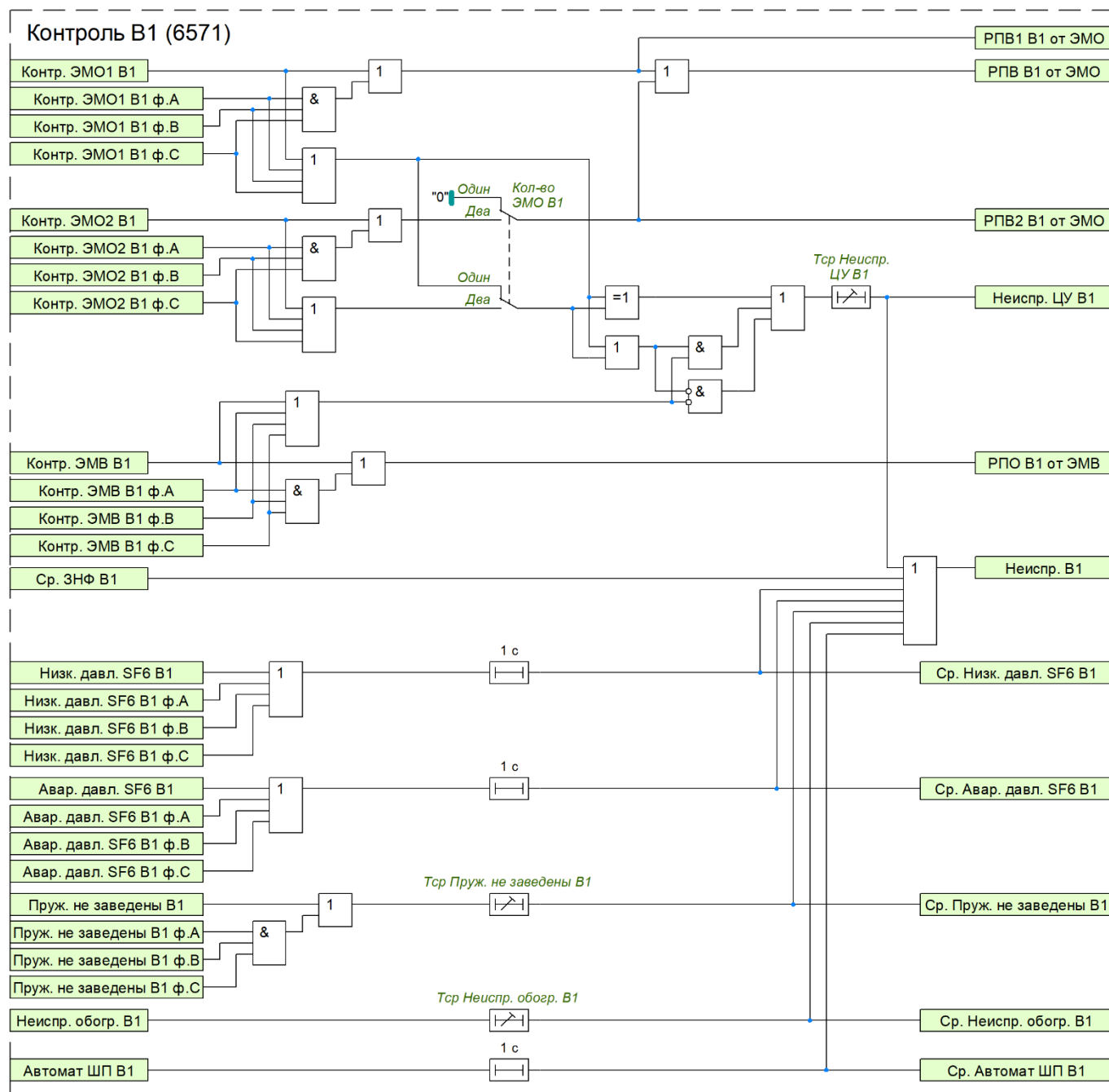
Рисунок 47 – Функциональная схема контроля В1
