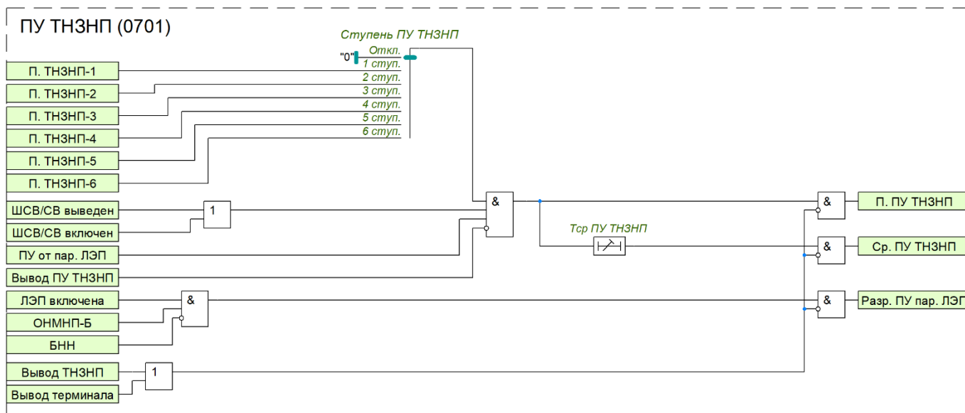
Рисунок 23 – Функциональная схема пуска ПУ ТНЗНП
