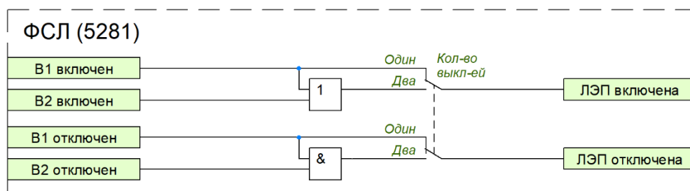
Рисунок 55 – Функциональная схема ФСЛ
