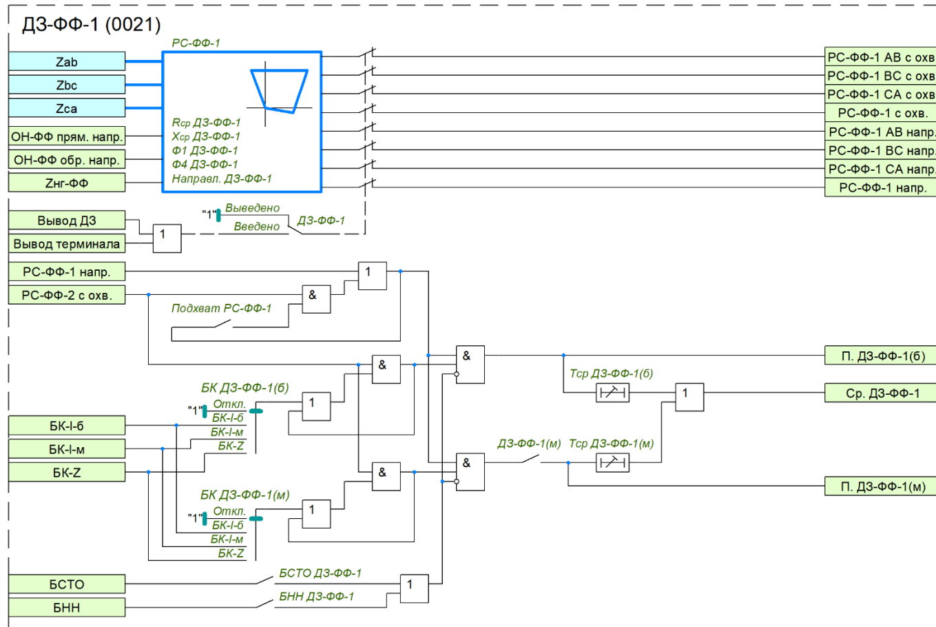
Рисунок 7 – Функциональная схема ДЗ-ФФ-1
