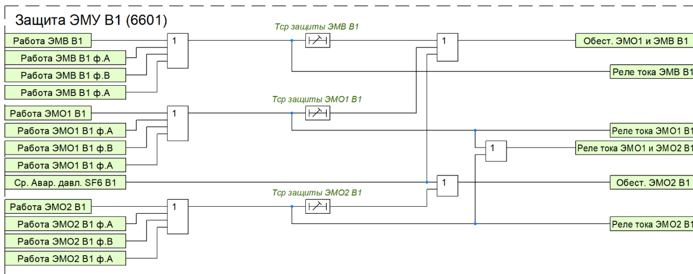
Рисунок 50 – Функциональная схема защиты ЭМУ В1
