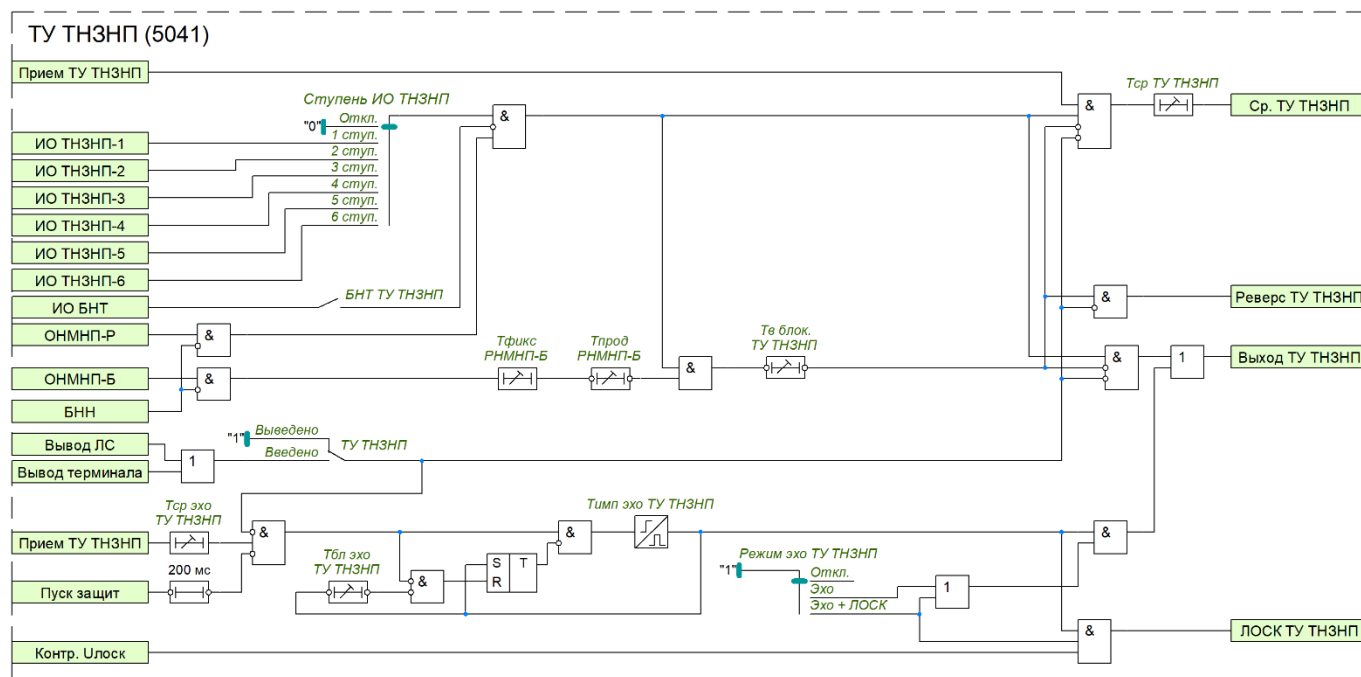
Рисунок 39 – Функциональная схема ТУ ТНЗНП
