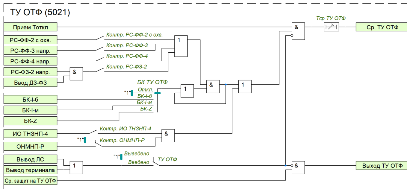
Рисунок 35 – Функциональная схема ТУ ОТФ
