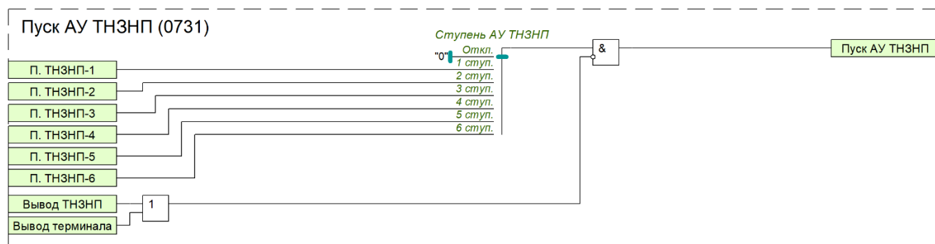
Рисунок 20 – Функциональная схема пуска АУ ТНЗНП
