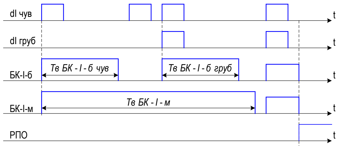
Рисунок 16 – Временная диаграмма работы БК-I
