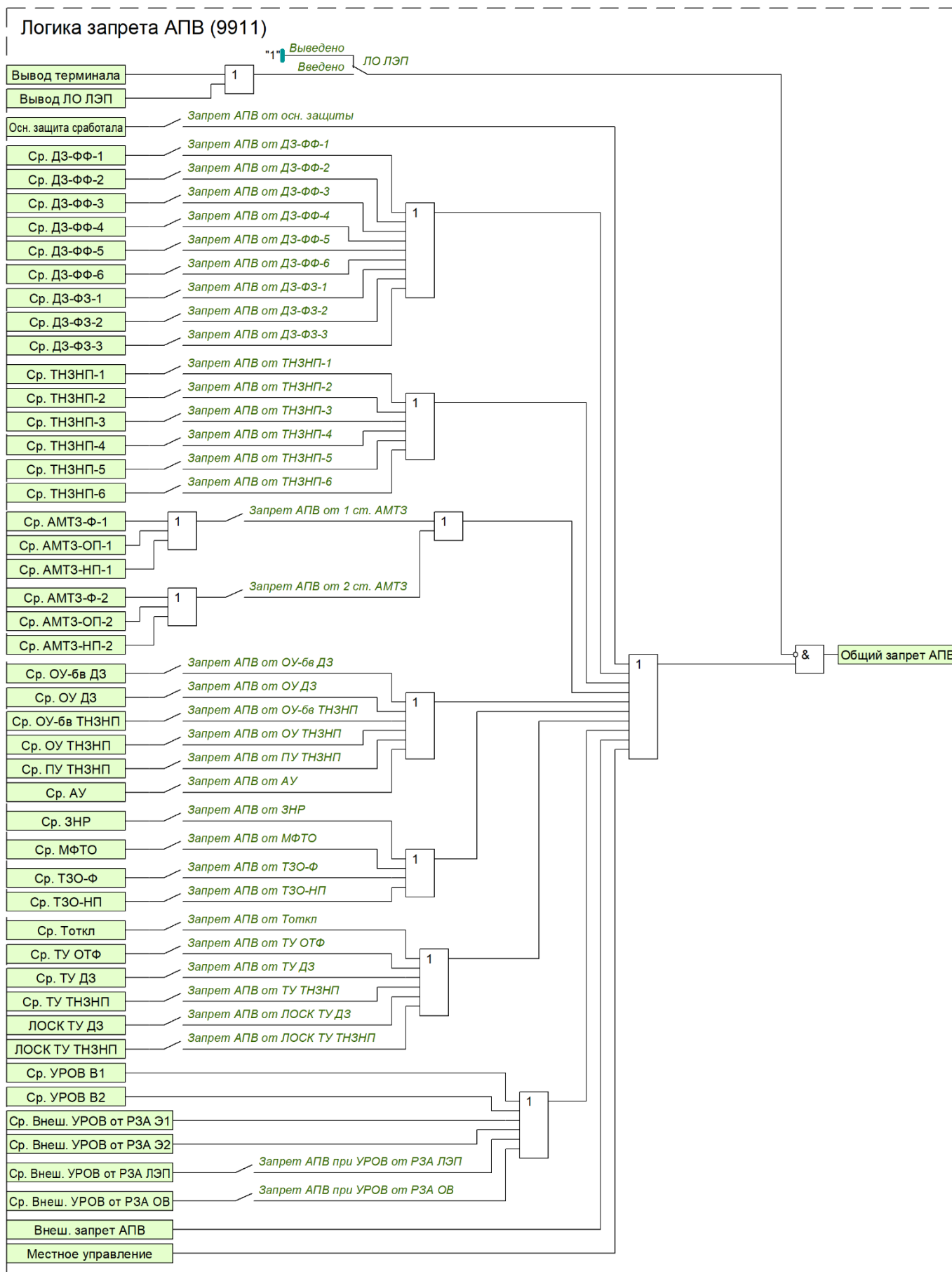
Рисунок 44 – Функциональная схема общего запрета АПВ
