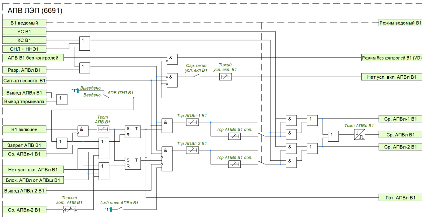
Рисунок 42 – Функциональная схема АПВ ЛЭП В1
