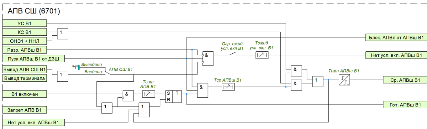
Рисунок 43 – Функциональная схема АПВ СШ В1
