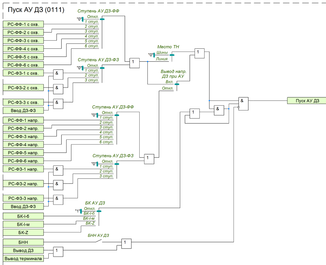
Рисунок 12 – Функциональная схема пуска АУ ДЗ
