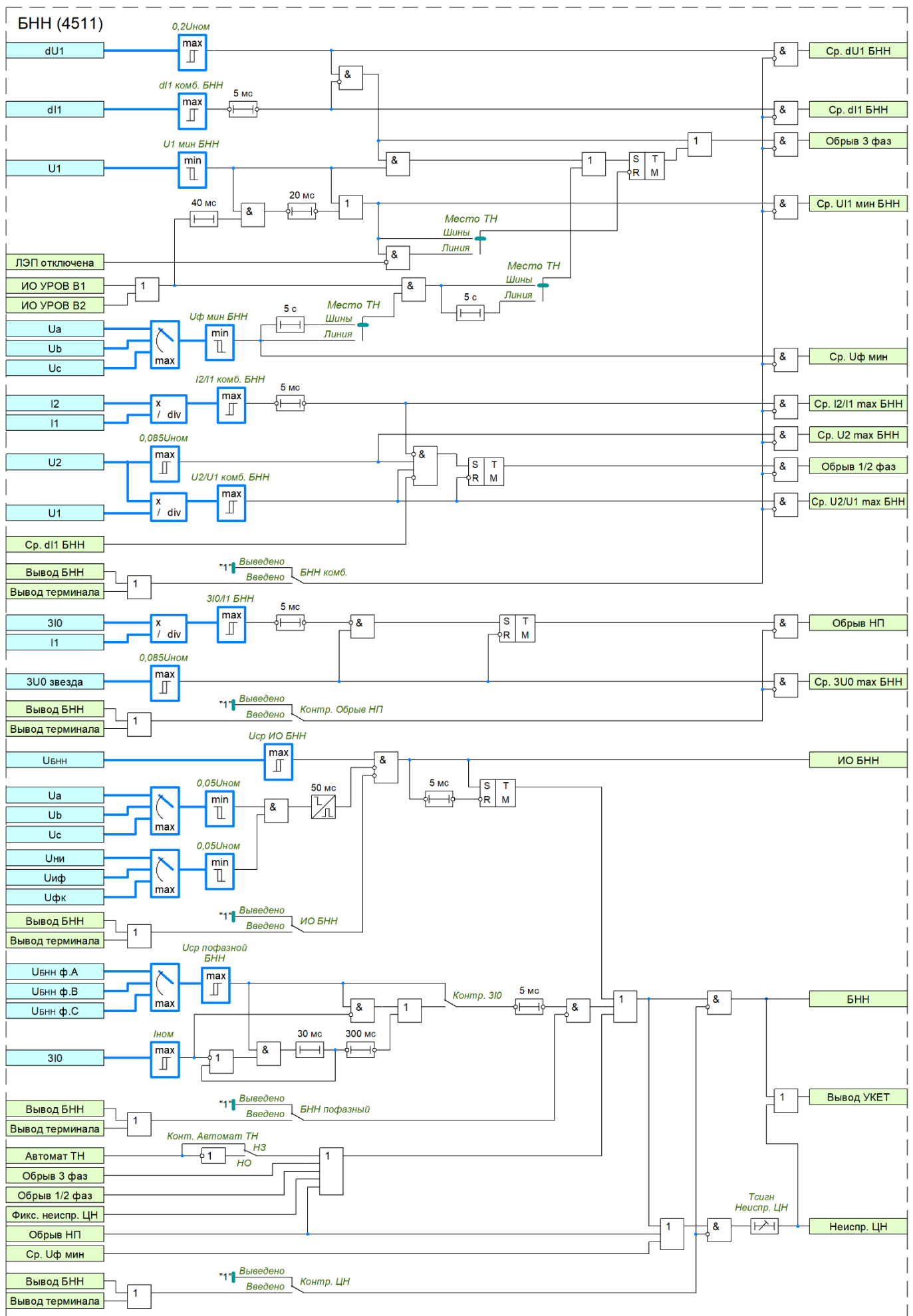
Рисунок 32 – Функциональная схема БНН
