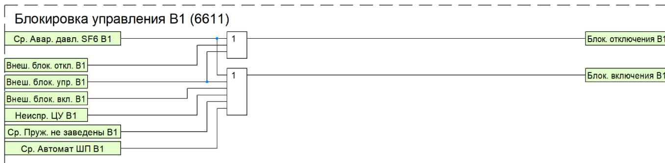
Рисунок 51 – Функциональная схема блокировки управления В1
