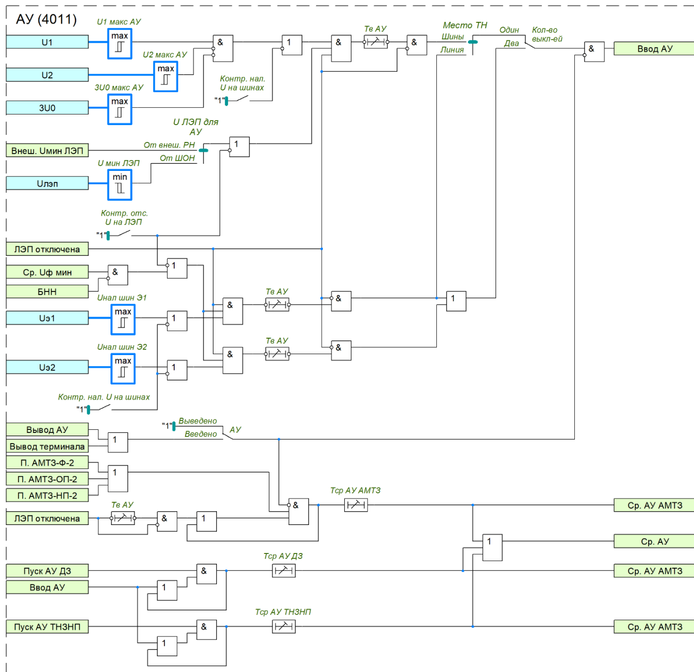
Рисунок 33 – Функциональная схема АУ
