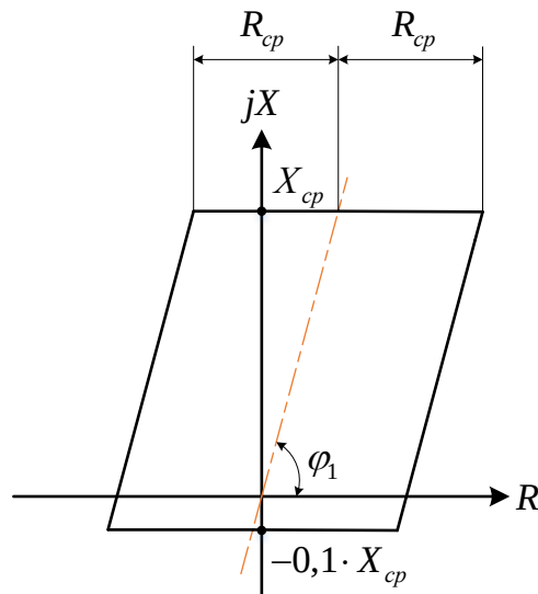
Рисунок 5 – Характеристика срабатывания направленного РС с охватом начала координат
