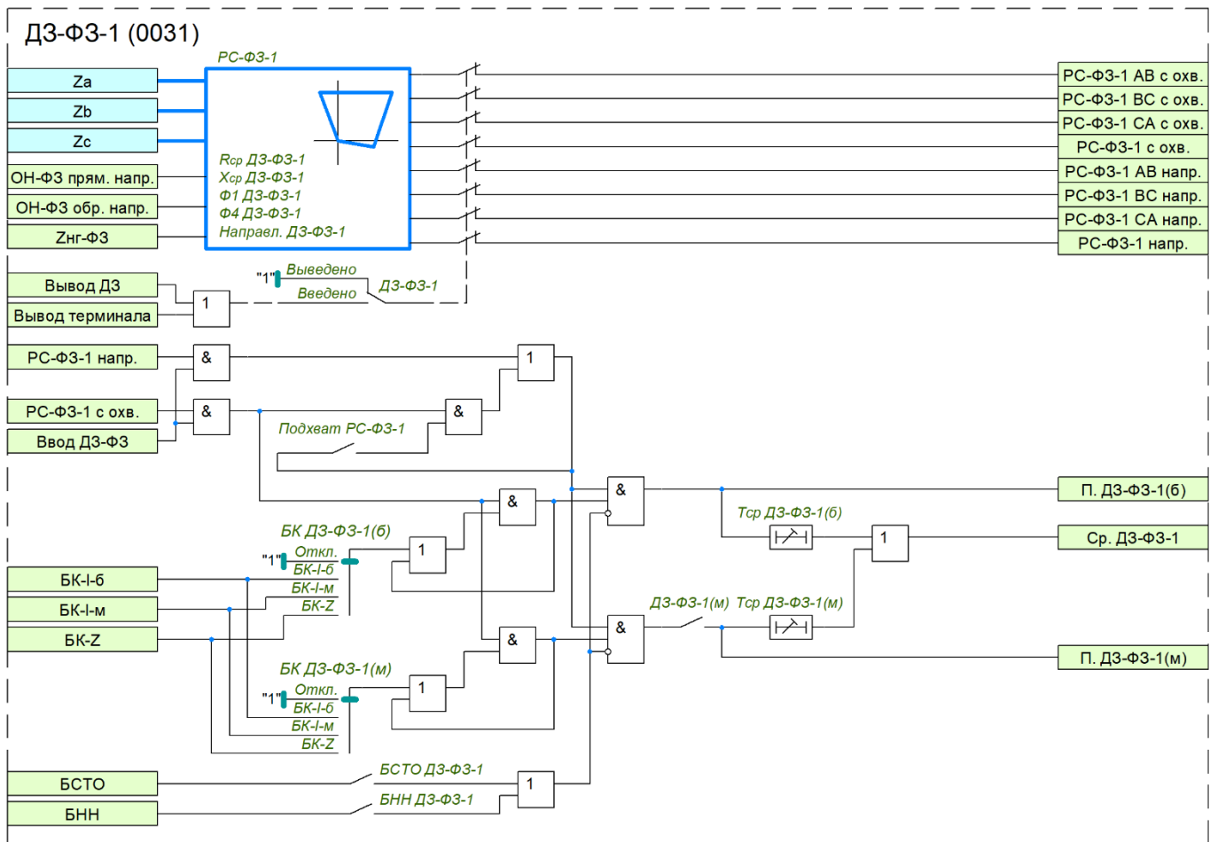
Рисунок 10 – Функциональная схема ДЗ-ФЗ-1
