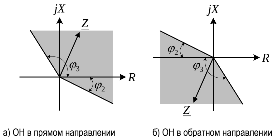
Рисунок 2 – Характеристики срабатывания органов направления
