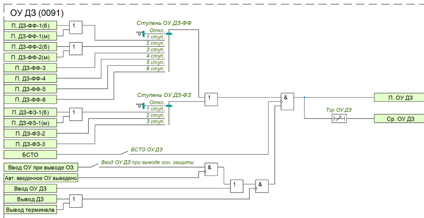
Рисунок 13 – Функциональная схема ОУ ДЗ
