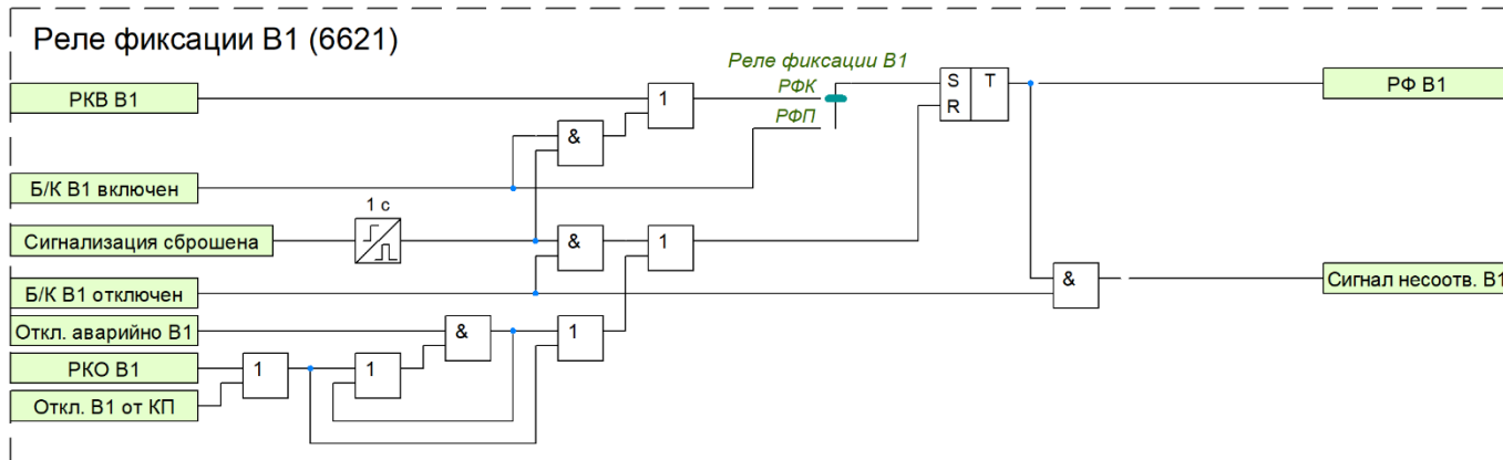
Рисунок 52 – Функциональная схема реле фиксации В1
