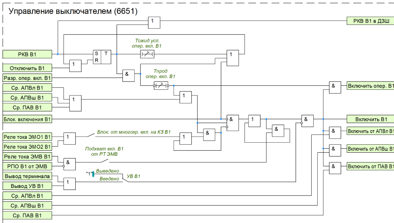
Рисунок 54 – Функциональная схема управления выключателем В1
