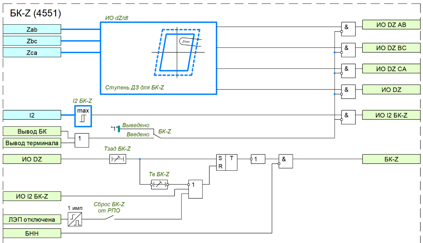
Рисунок 17 – Функциональная схема БК-Z
