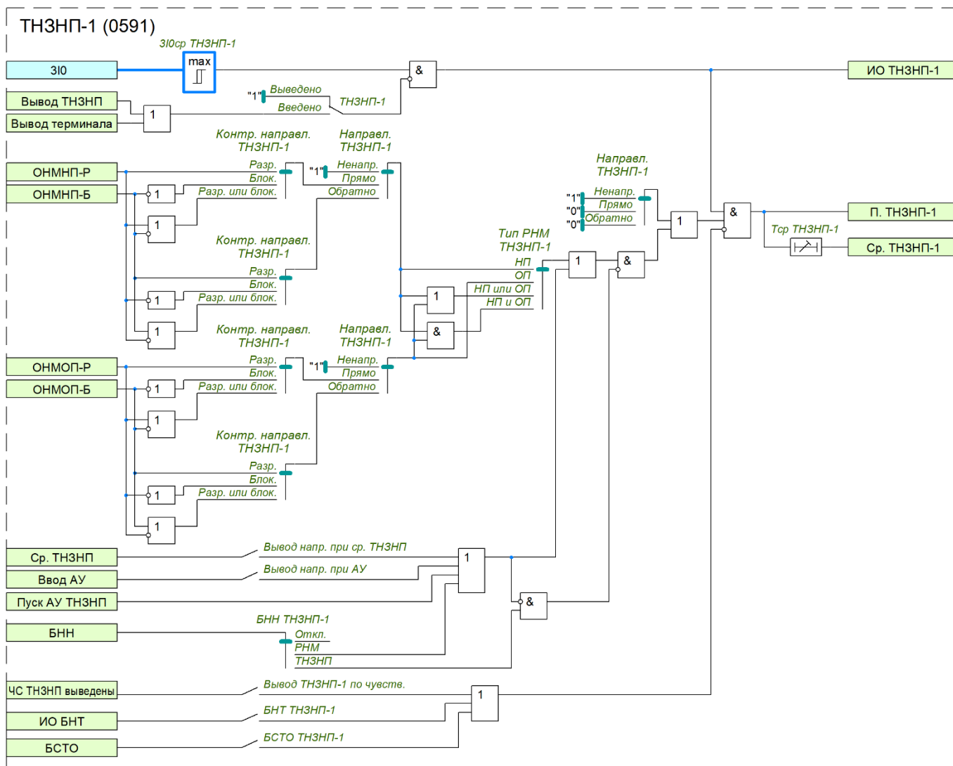
Рисунок 24 – Функциональная схема ступени TN3NP
