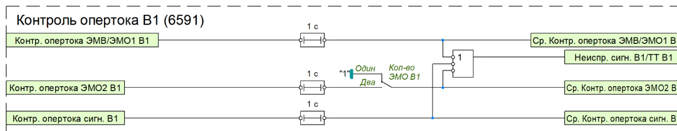
Рисунок 49 – Функциональная схема контроля опертока В1
