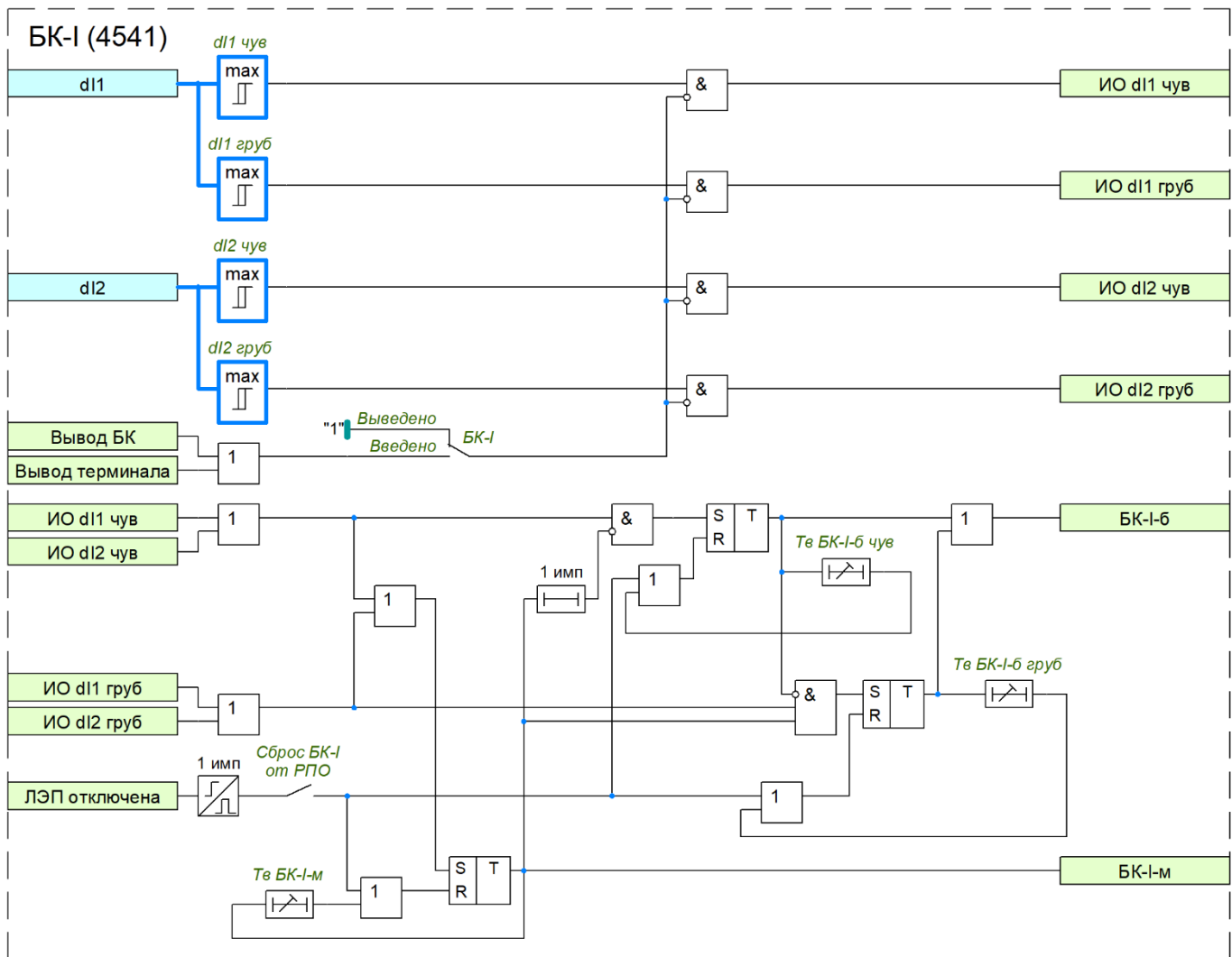
Рисунок 15 – Функциональная схема БК-I
