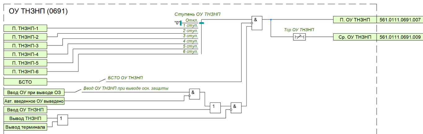
Рисунок 21 – Функциональная схема ОУ ТНЗНП
