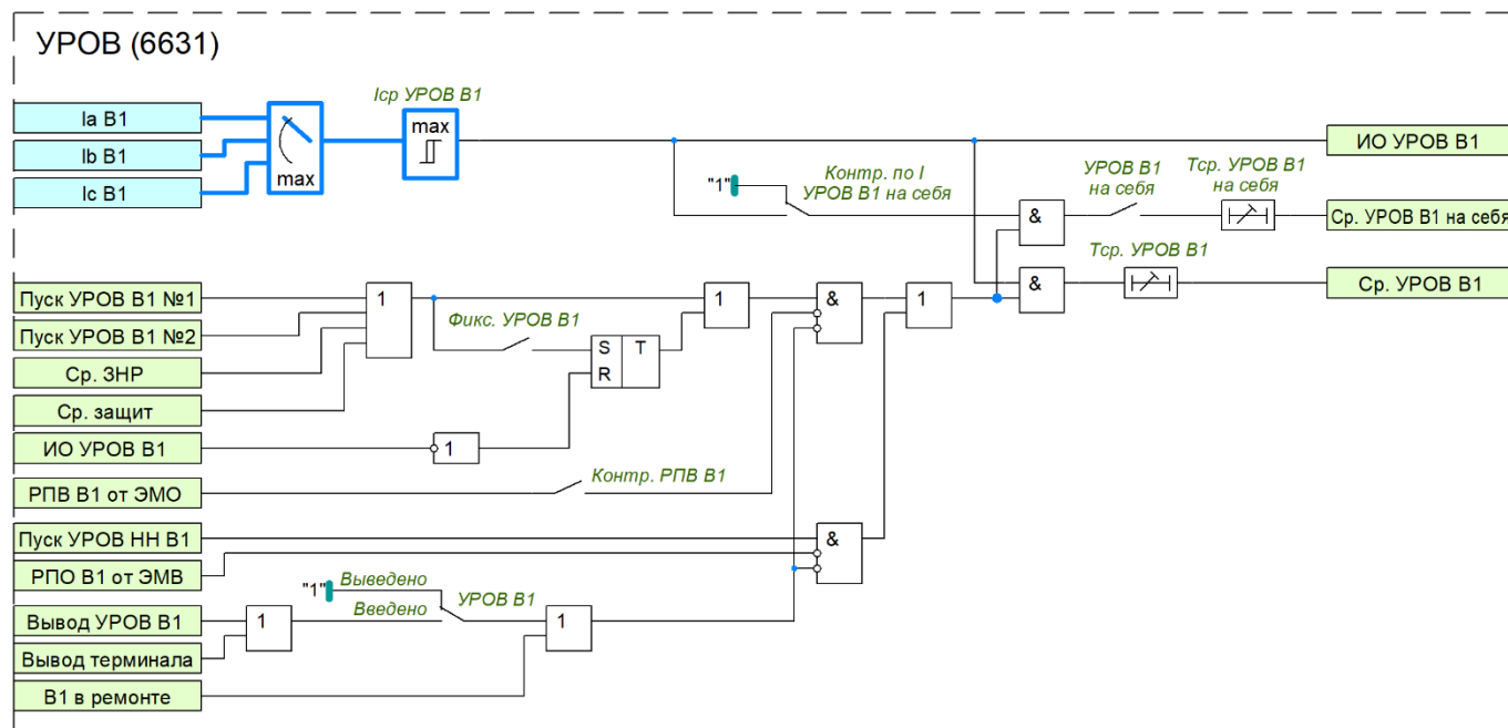
Рисунок 40 – Функциональная схема УРОВ В1
