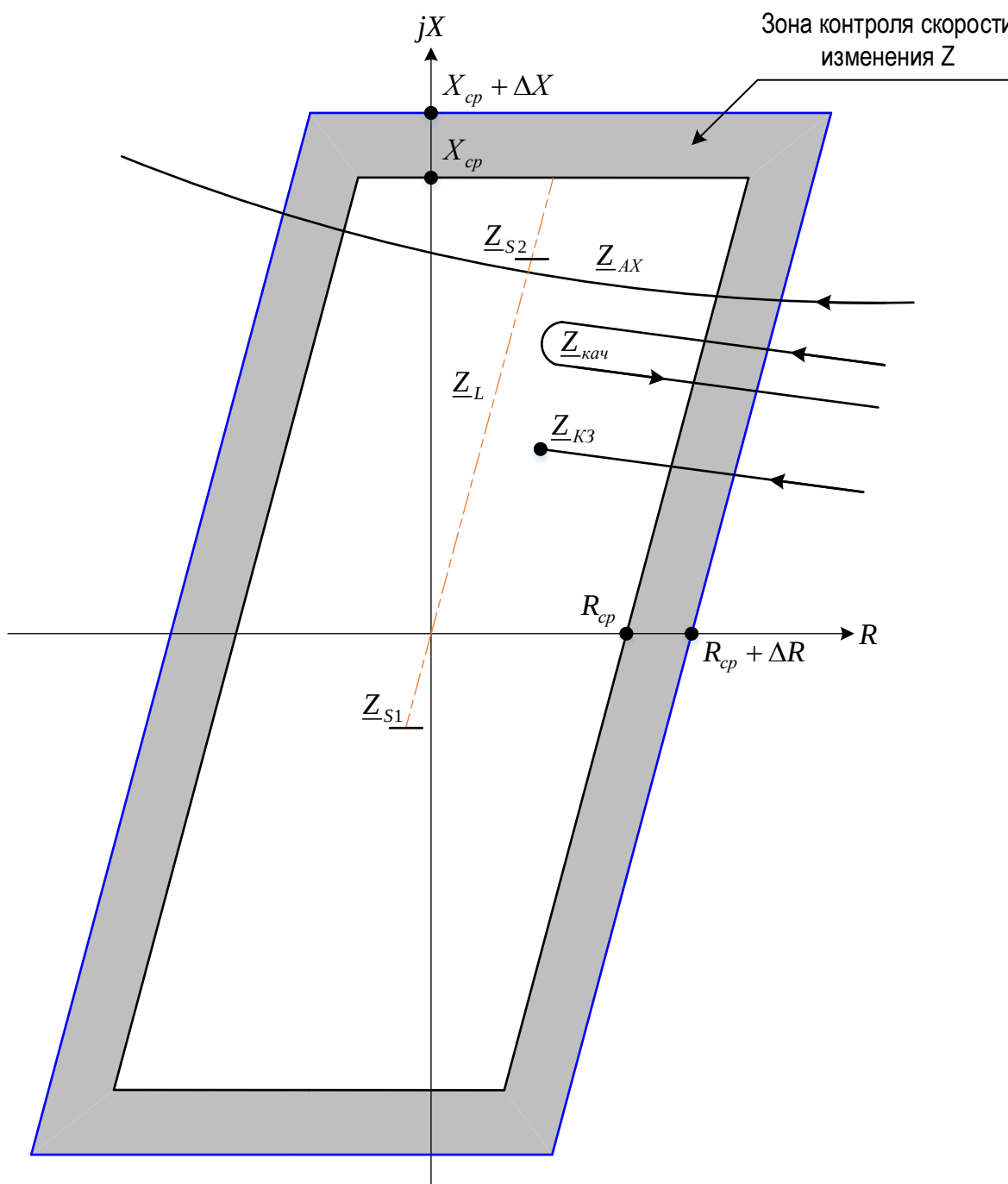
Рисунок 18 – Характеристики реле сопротивления, используемые для блокировки при качаниях по скорости изменения сопротивления
