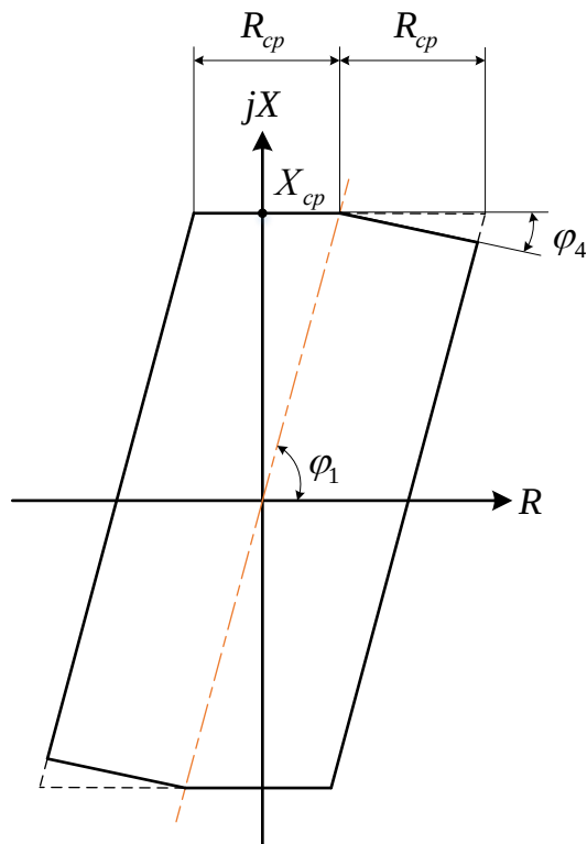
Рисунок 1 – Характеристика срабатывания ненаправленного РС
