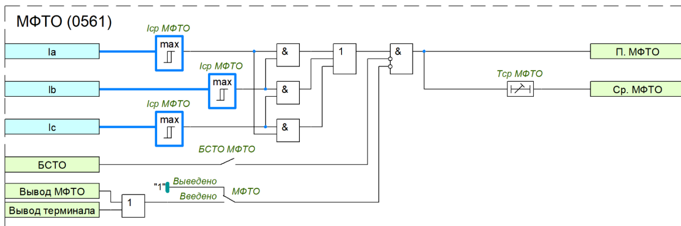
Рисунок 25 – Функциональная схема МФТО
