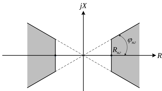
Рисунок 3 – Характеристика срабатывания измерительного органа отстройки от нагрузки
